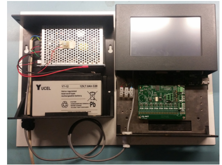
备用电池和FG-NET数字主机之间的连接示例
