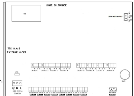
FG-ALS8-0D 线路图
