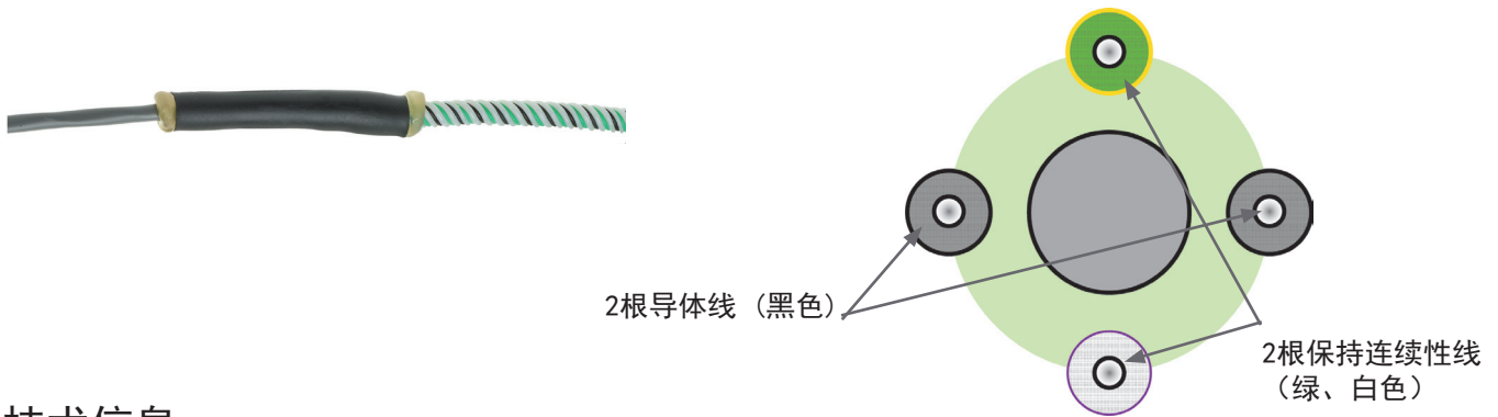
FG-ACS 4芯酸液检测线缆横切面
