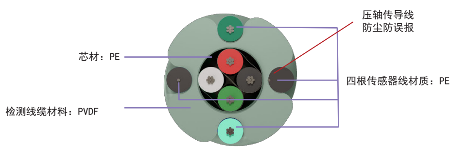
FG-AC 检测线缆切割视图
